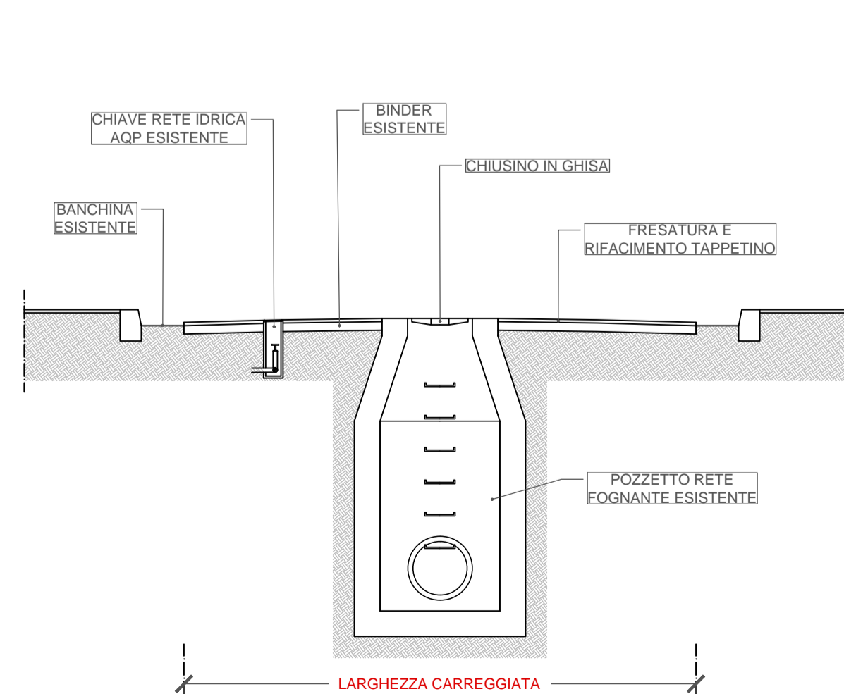
DETTAGLIO INTERVENTO DI FRESATURA E RIPRISTINO DEL MANTO STRADALE_SCALE 1:50
