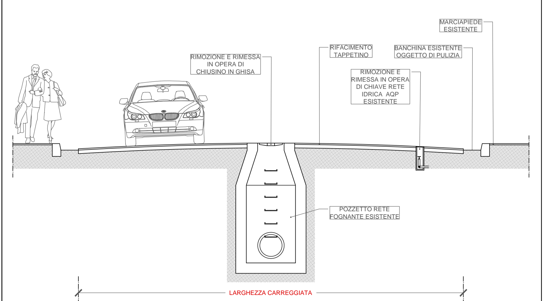
DETTAGLIO INTERVENTO RIPRISTINO DEL MANTO STRADALE_SCALE 1:50
